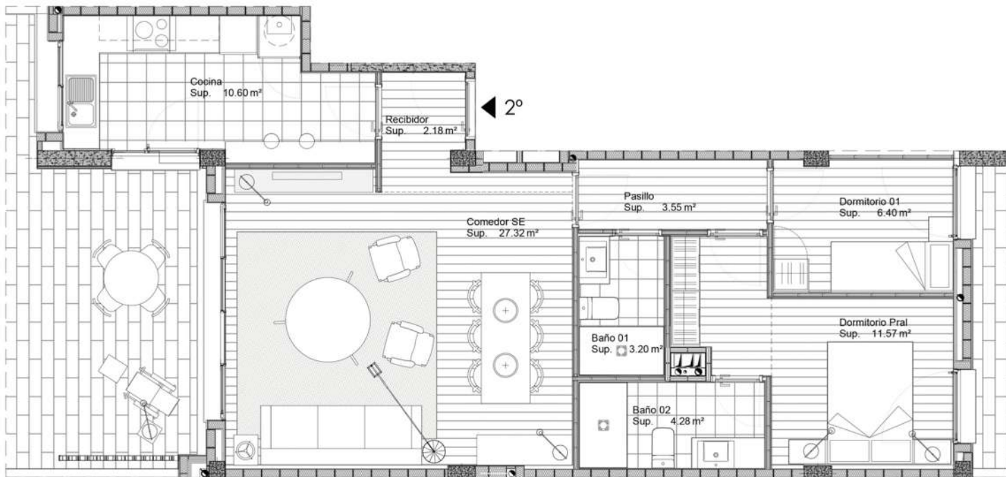
Esc. A- Planta 02 TIPO T2a
